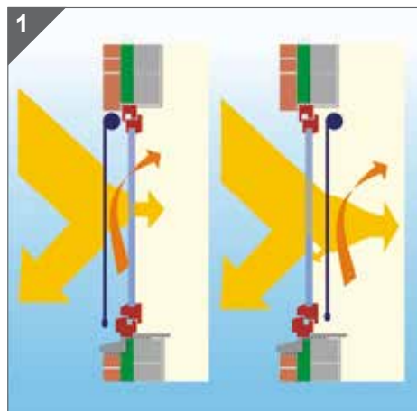
Comportamiento del sombreado solar en relación al calor, según su posición.
