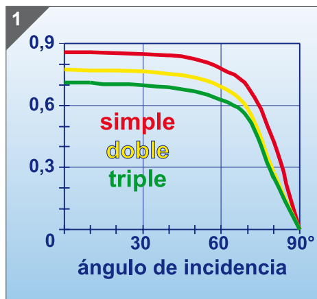
Variaciones en el factor solar en función del ángulo de incidencia de los rayos de Sol.
