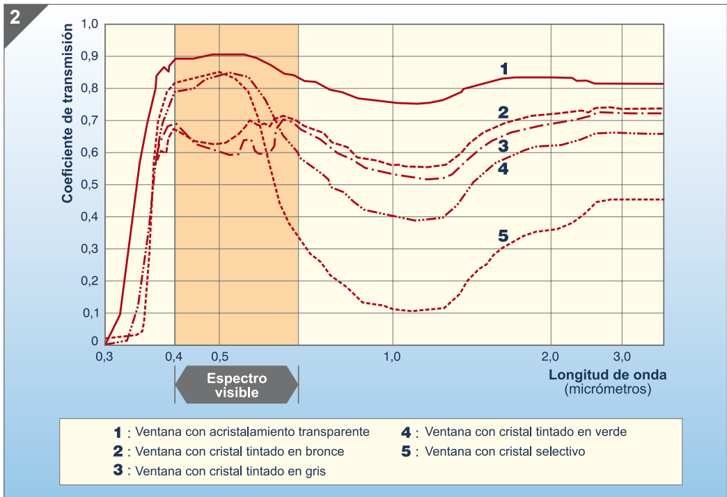
Curvas que representan la transmisión de la luz espectral de varios acristalamientos tintados.
