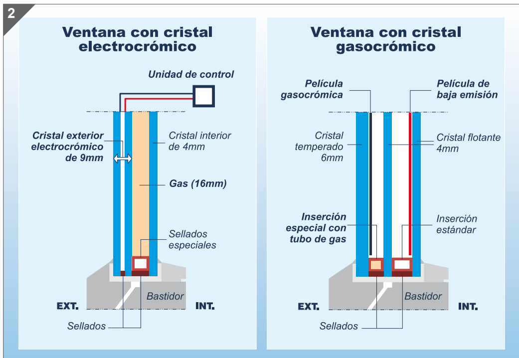
a: Funcionamiento del acristalamiento electrocrómico. b: Funcionamiento del acristalamiento gasocrómico.
