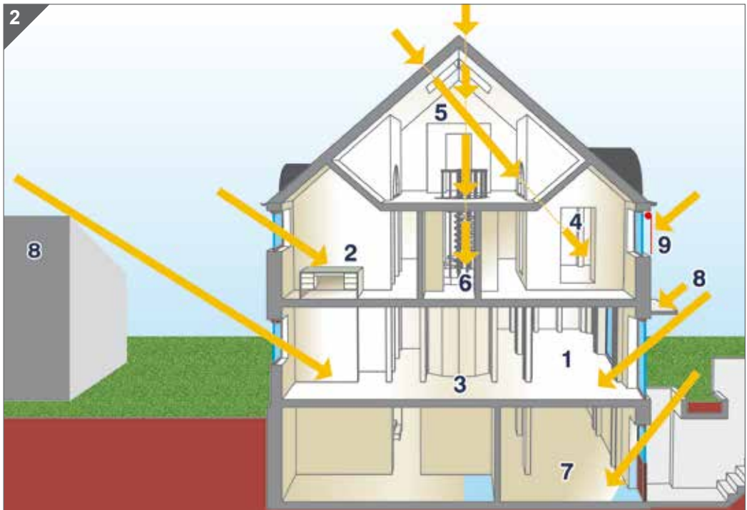
Conceptos de iluminación natural para una vivienda unifamiliar.
