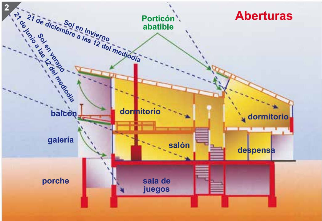
El estudio de una sección transversal de los huecos de un edificio permite determinar los niveles y el calendario de la luz del día y el aporte solar. (arquitecto: H. Bolliger).
