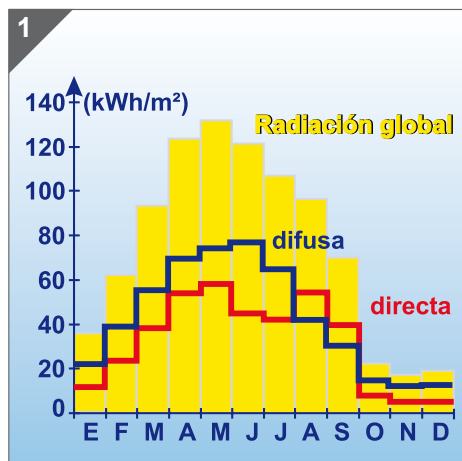
Energía promedio recibida sobre una superficie horizontal en Bruselas.
