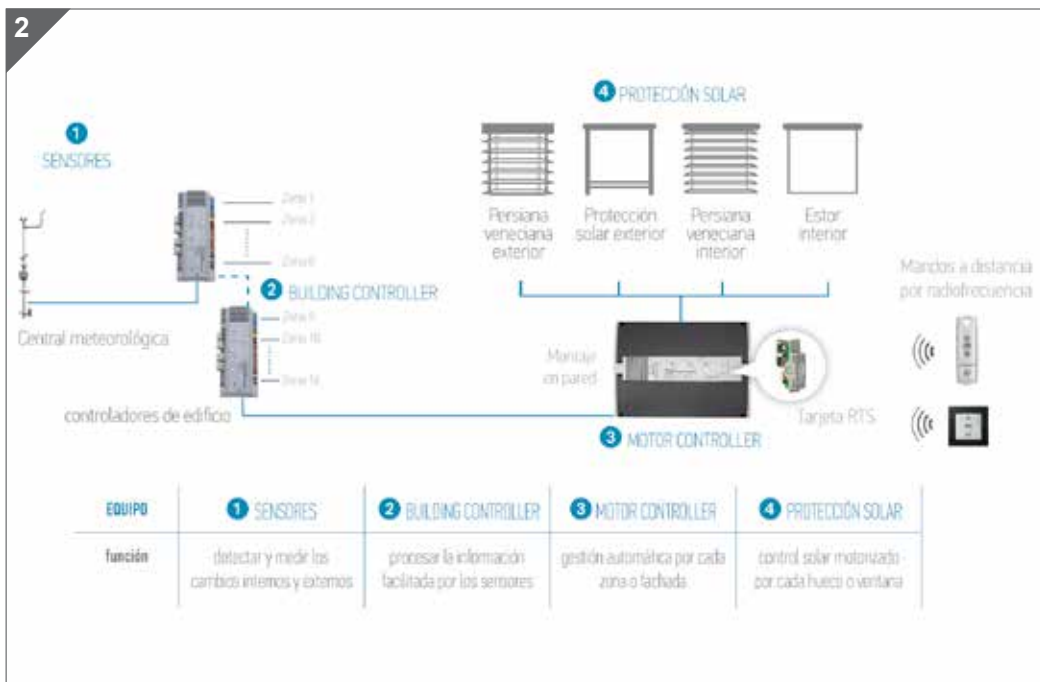
Sun Tracking en 4 pasos: 1 Sensores. 2. BuCo, 3 MoCo, 4 Protección Solar
