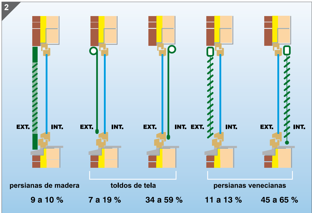
Factores solares para diferentes tipos de protección solar con acristalamiento simple.
