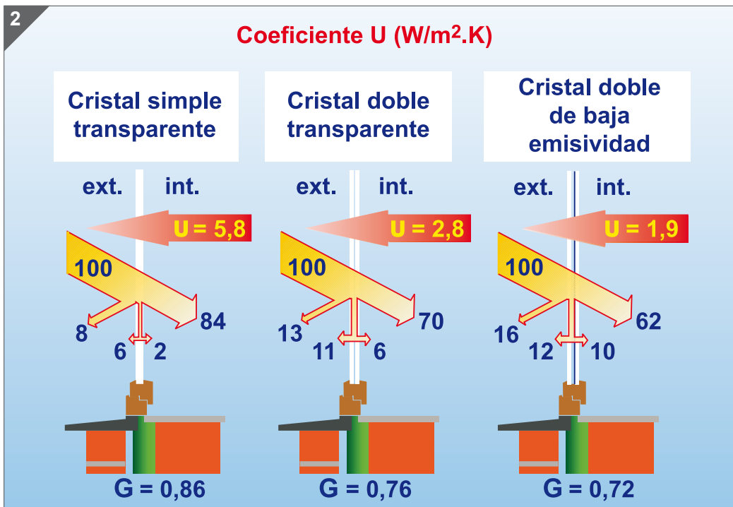
Comportamiento térmico de los diferentes tipos de acristalamiento.
