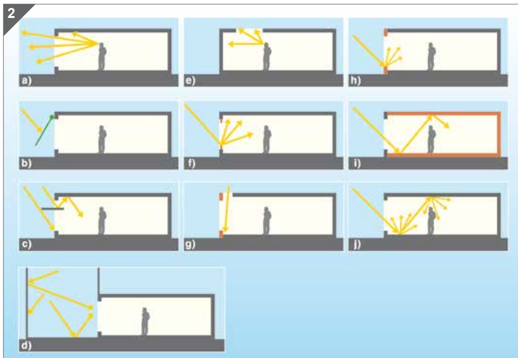
Reducción del deslumbramiento gracias a la luz natural.
