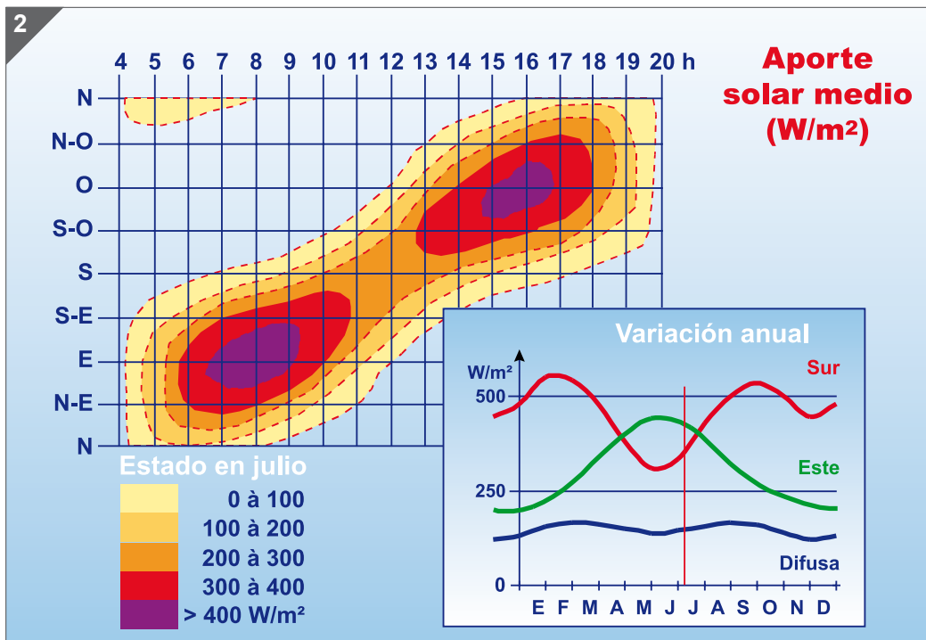
Energía promedio recibida sobre una superficie vertical en Carpentras (Francia).
