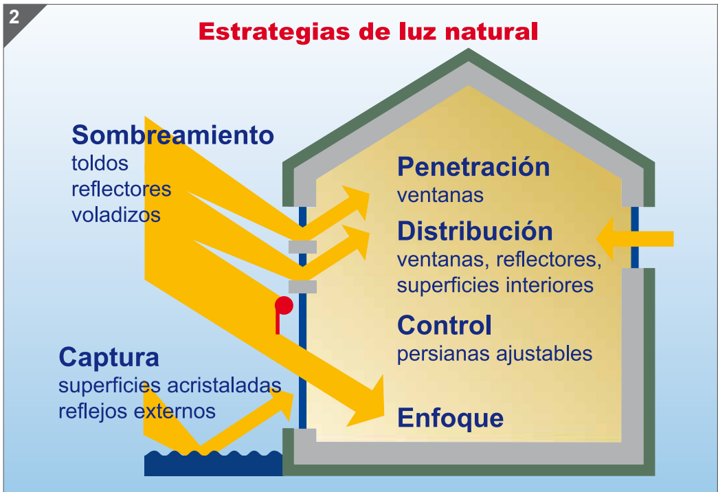
Estrategias para el control de la luz natural.
