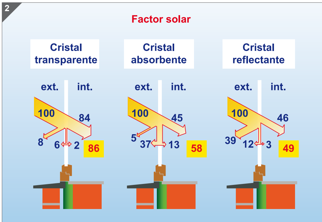
Factores solares para acristalamientos simples y ángulos de incidencia específicos.
