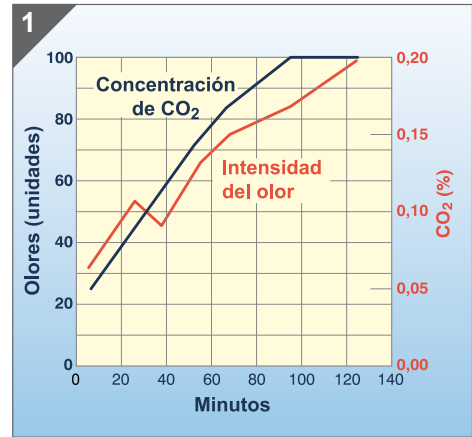
Incremento paralelo de las concentraciones de CO 2 y la intensidad de los olores.
