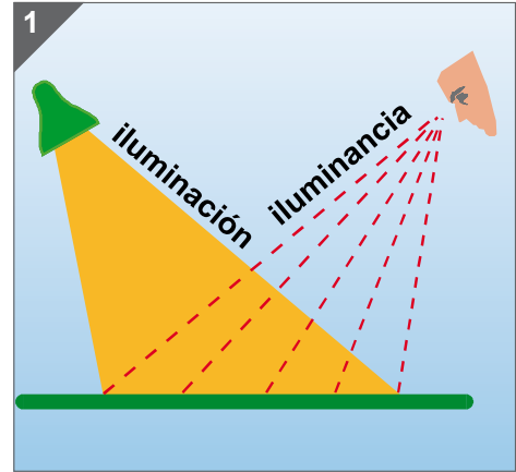
La percepción de la iluminancia depende de la iluminación y del índice de refracción de una superficie.
