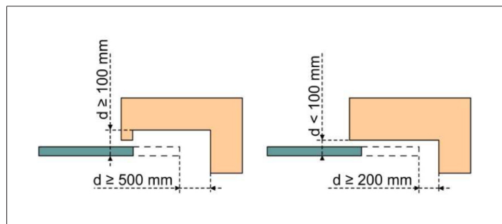
Slika 2: Bezbedna udaljenost
